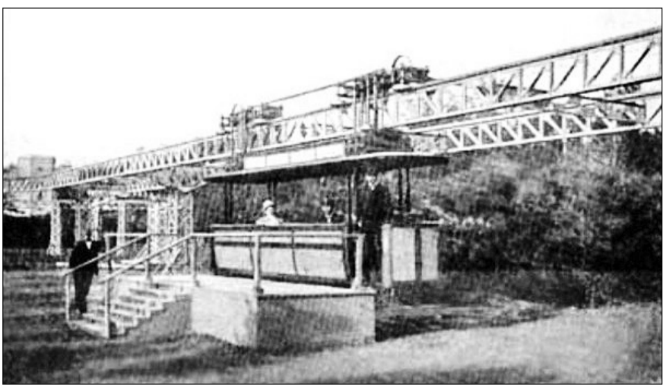
Подвесная электрическая дорога. Инженер – Ипполит Владимирович Романов. Гатчина, июнь 1900 г.
